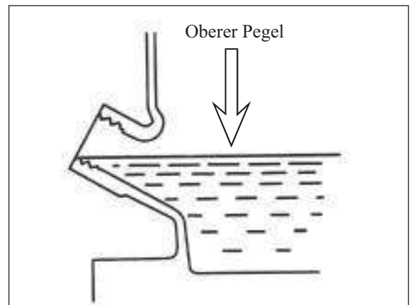
Öleinfüllverschluß beim Honda GX-Motor.
