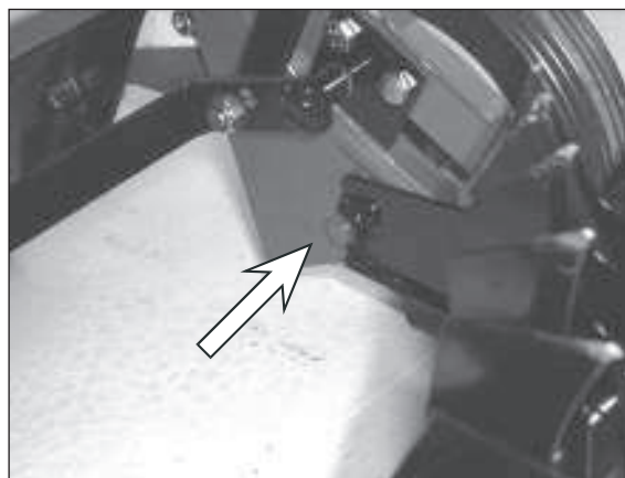
2) Montagehinweis: Achten Sie darauf, dass der Zapfen in der Aufnahme steckt.
