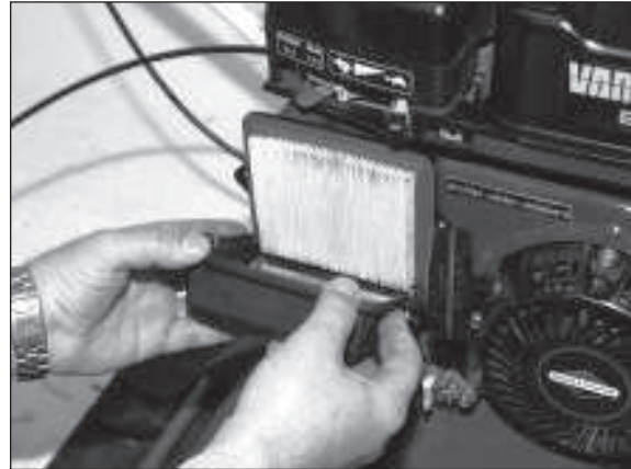
2) Deckel abnehmen.
