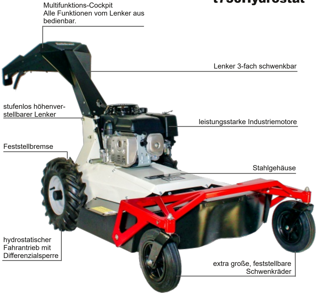
Abb. zeigt t750Hydrostat
